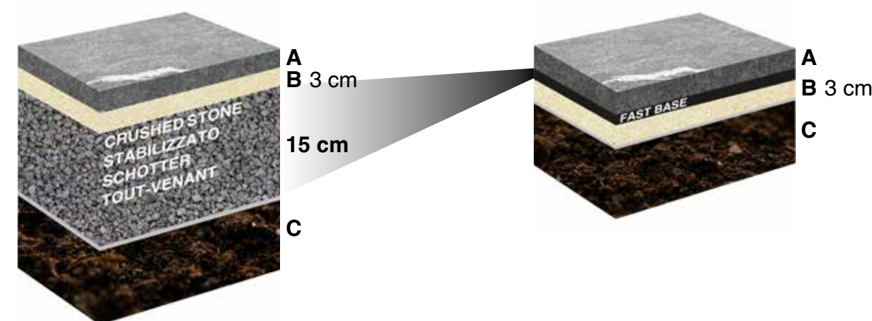
3 Posizionare FAST BASE e tagliarlo sul perimetro Position FAST BASE and cut it on the perimeter Positionieren Sie Fast Base und schneiden Sie die Enden zu. Positionner FAST BASE et découper-le sur le périmètre
